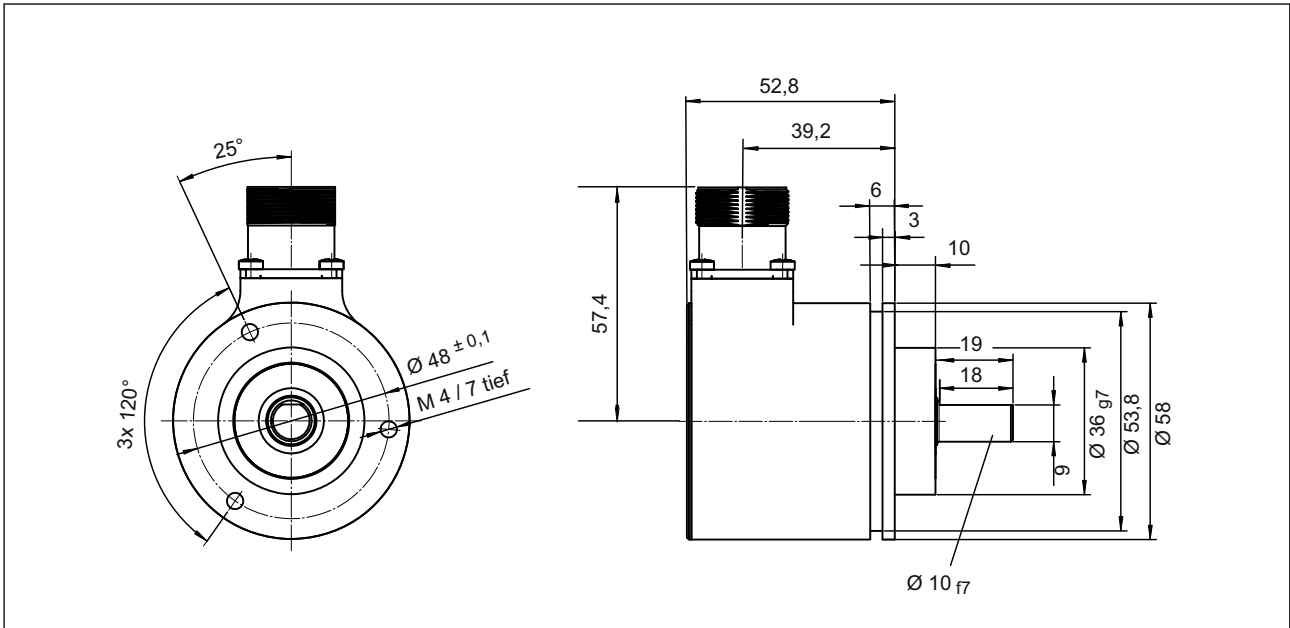
Maßbild GEL 2037 – Klemmflansch mit Zahnradadapter
