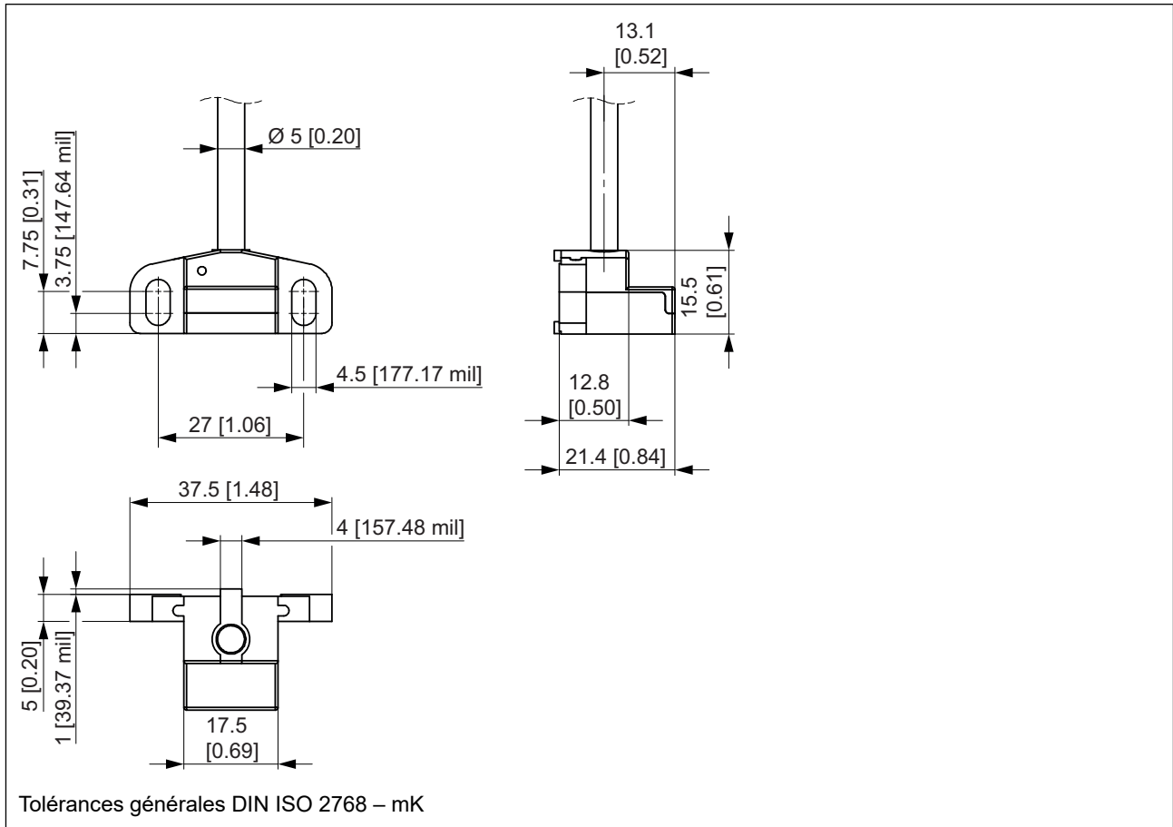
Dessin coté sortie de câble MiniCODER (T) — tangentielle, sortie de câble à droite
