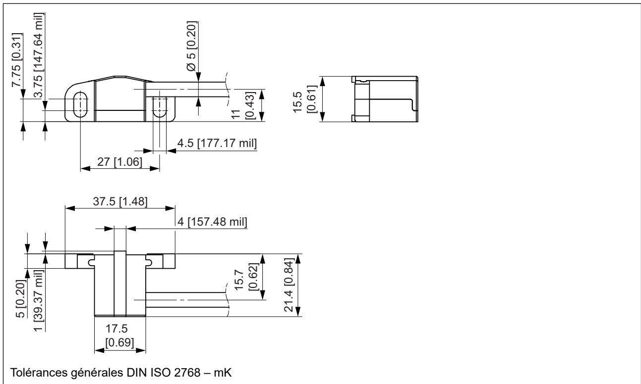
Dessin coté sortie de câble MiniCODER (T) — tangentielle, sortie de câble à droite
