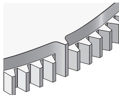
Z = marque de référence – dent Roue dentée de mesure standard
